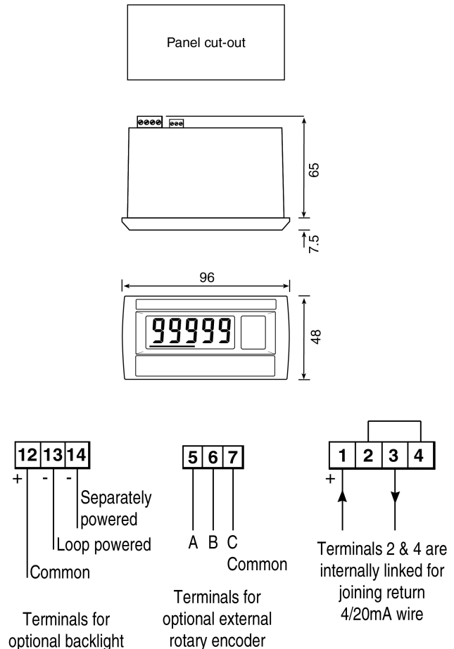
Fig 4 BA427E dimensions
